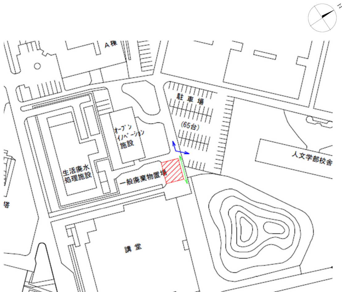
オープンイノベーション施設付近 配置図
