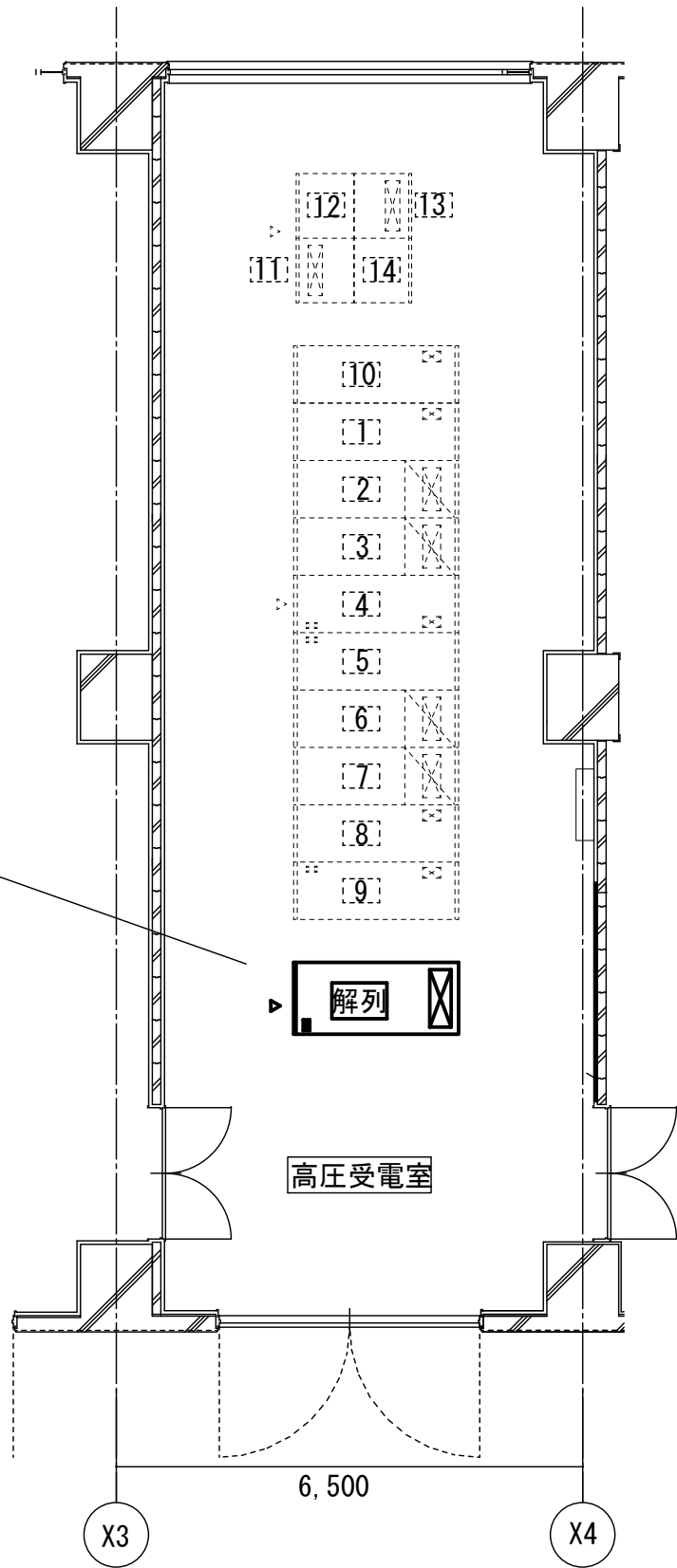
エネルギーセンター2階平面図（高圧受電室） S=1/100
