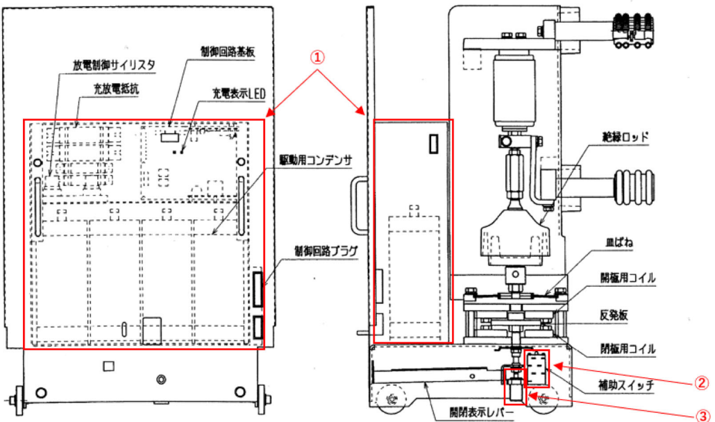
6-HSS-20 形高速真空遮断器(VCB)交換部品
