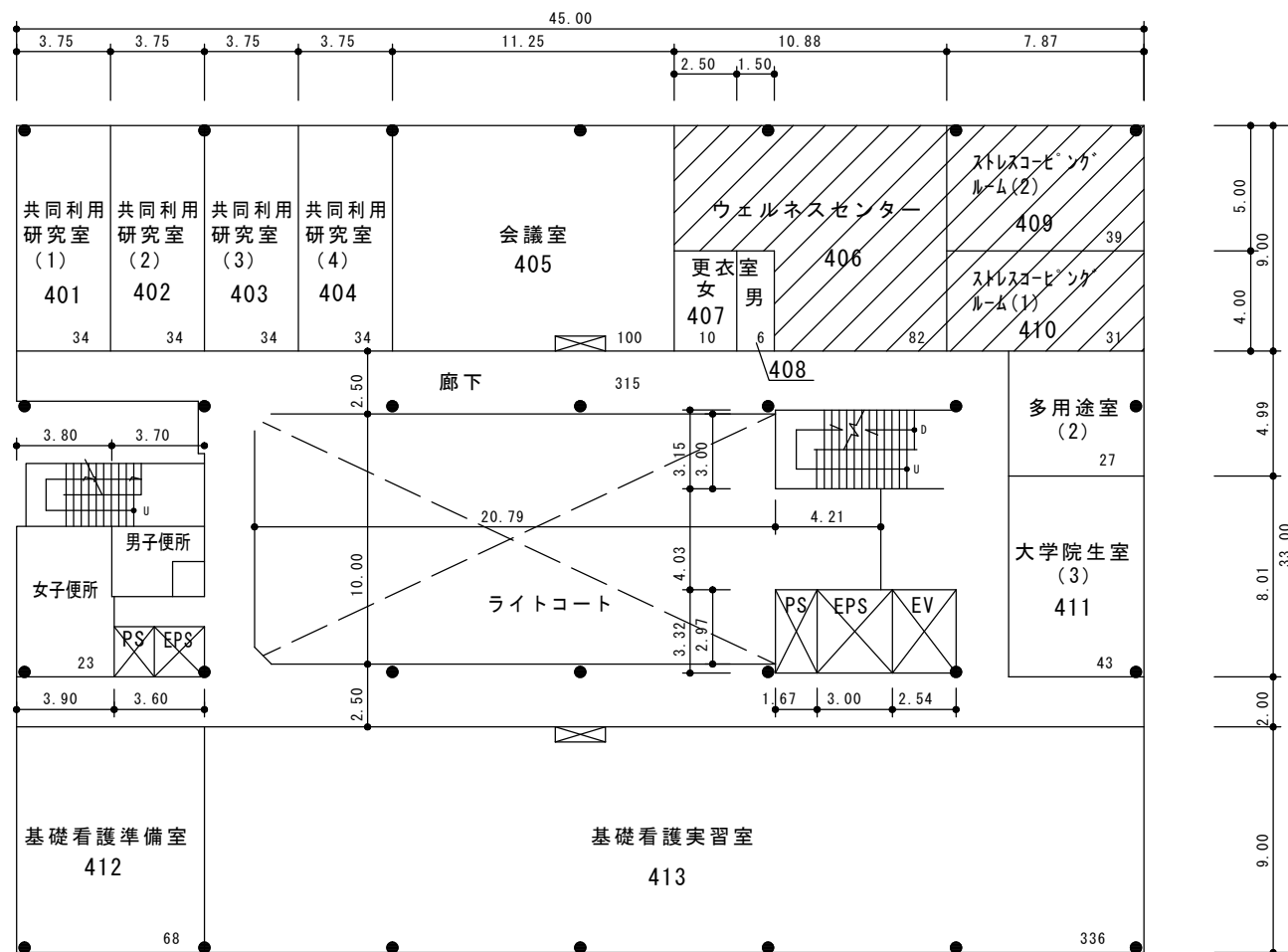
看護学科棟 4階平面図
