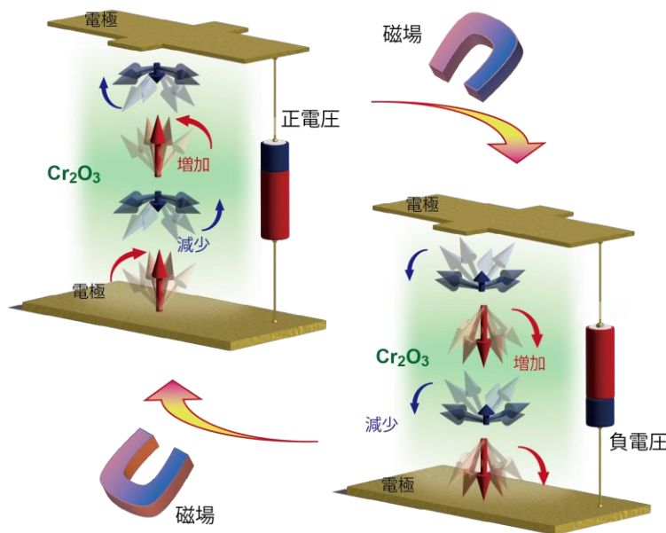
(a) クロム酸化物を用いたデバイスの模式図
