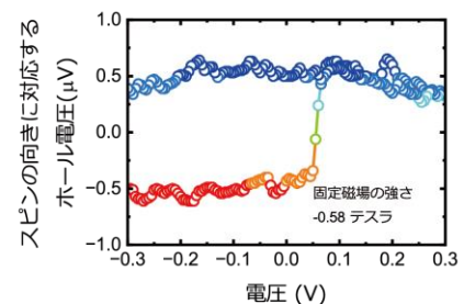
(c) スピン反転の電圧(電界)による変調
