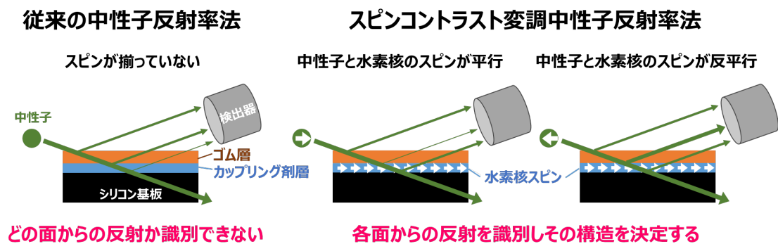
図 2 従来の中性子反射率法とスピンコントラスト変調中性子反射率法の比較
