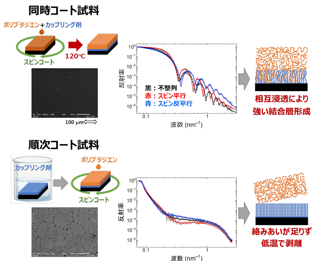
図 3 ポリブタジエン/シランカップリング剤の同時・順次コート薄膜試料の SEM 画像(左)、中性子反射率曲線(中央)、測定から決定された薄膜の構造(右)
