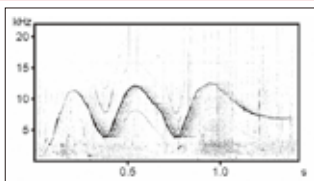
図2 ホイッスル(ピュイピュイピュイと聞こえる)の音響スペクトログラム。縦軸が音の高さ(周波数; kHz)、横軸が時間(秒; s)
