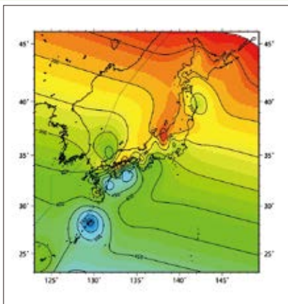
「120年に1回」起これる豪雨(日降水量)の等値線図(陸上だけ見てください)
