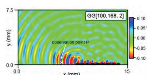
▲ 高指向性テラヘルツ電磁波放射
