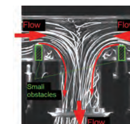
▲ 小物体による T字合流管内の流動制御
