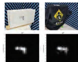
▲ ミリ波を用いた非接触イメージング
