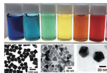
▲ 様々な形の金属ナノ粒子の電子顕微鏡像とその分散液の色
