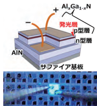
▲窒化物半導体による青色LED
