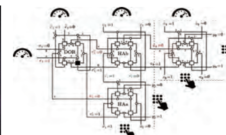
▲ 量子素子回路の例
