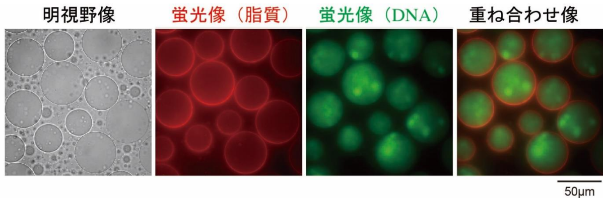
図3：リン脂質の膜で区画化・小胞化されたマイクロ液滴へのDNAの自発的なカプセル化。
