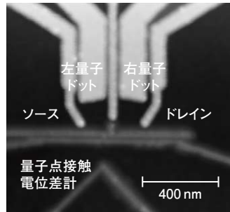
2重量子ドットおよびオンチップ量子点接触電位差計による単一電子実時間計数のセットアップ(スイス連邦工科大学との共同研究による)。(図2)
